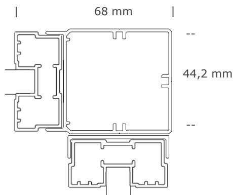
Søjle (hjørne)
