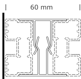
Startprofil mod væg
