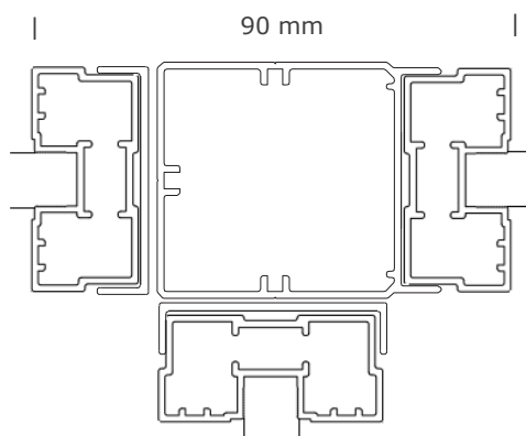
Søjle (T-løsning)
