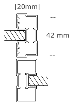
Overlap mellem skydedør og fast element
