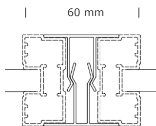
Clipsprofil
