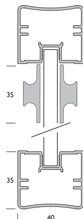
Skydedør med indvendigt greb, påklæbet (option)
