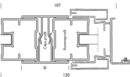
Dørramme med karm mellem 2 faste vægmoduler
