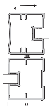
Skydedør med børstetætning (option)
