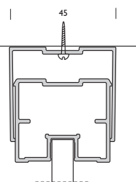
Startprofil mod væg
