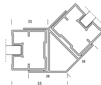
45° hjørneprofil
