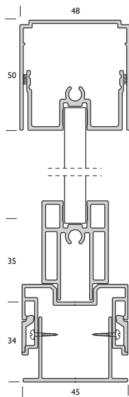
Eksempel på fast væg med justerbar sokkel
