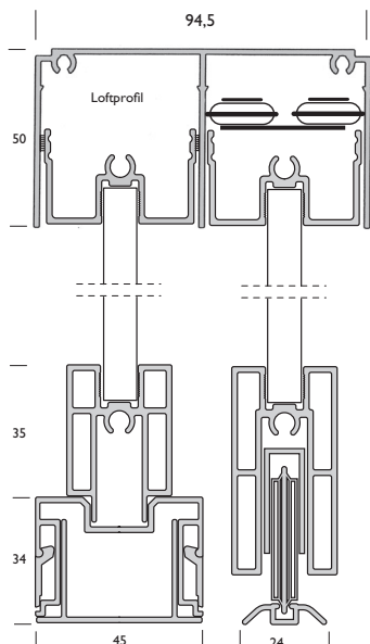
Dobbelt loftprofil
