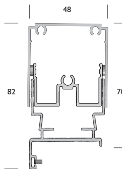
Overramme CUBE dør
