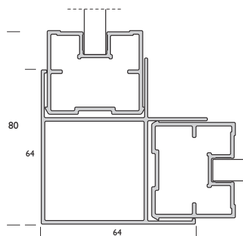
90° hjørneprofil
