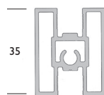
Sprosse til vandret deling af væg/dør
