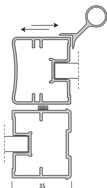
Skydedør med udvendigt greb (option)
