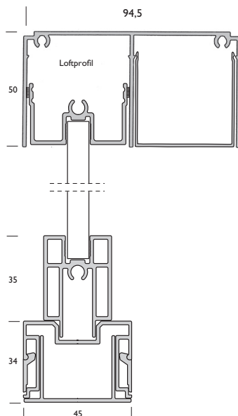
Dobbelt loftprofil med dæk profil
