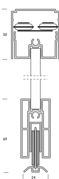
Skydedør med tophjul og justerbar bundhjul
