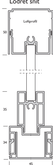
Fast væg med justerbar sokkel
