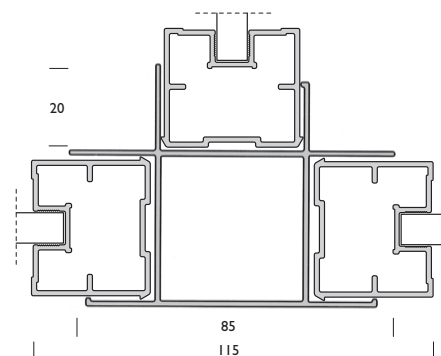
T-løsning
