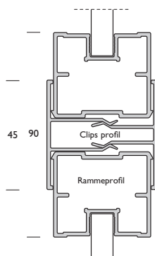
Clips profil
