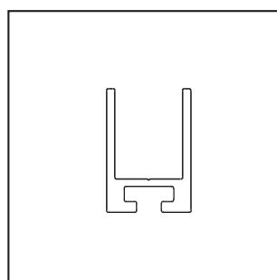
2_ Profil til gulv/væg 30 mm
